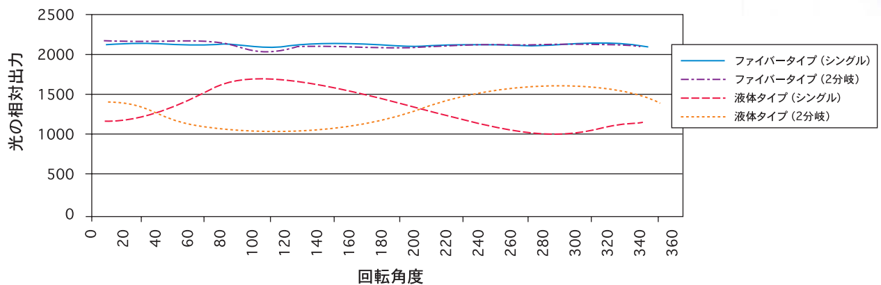
高出力ファイバライトガイドと、2分岐液体ライトガイドの光量比較
